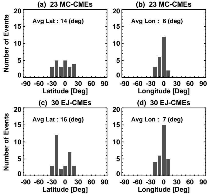
Figure 4. Histograms of the source locations: a) latitude and b) longitude for 23 MC-CMEs, c) latitude and d) longitude for 30 EJ-CMEs.
