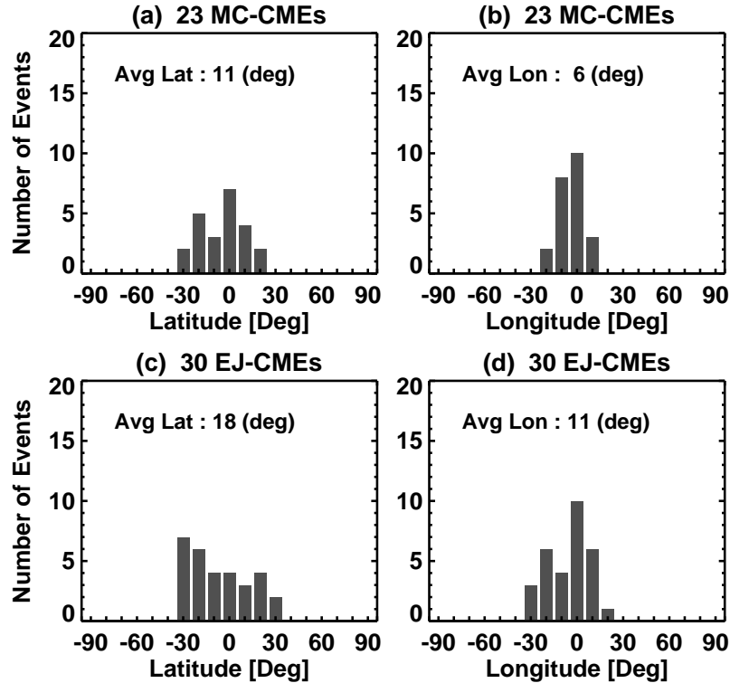
Figure 5. Histograms of the KFR-fit propagation directions: a) latitude and b) longitude for 23 MC-CMEs, c) latitude and d) longitude for 30 EJ-CMEs.
